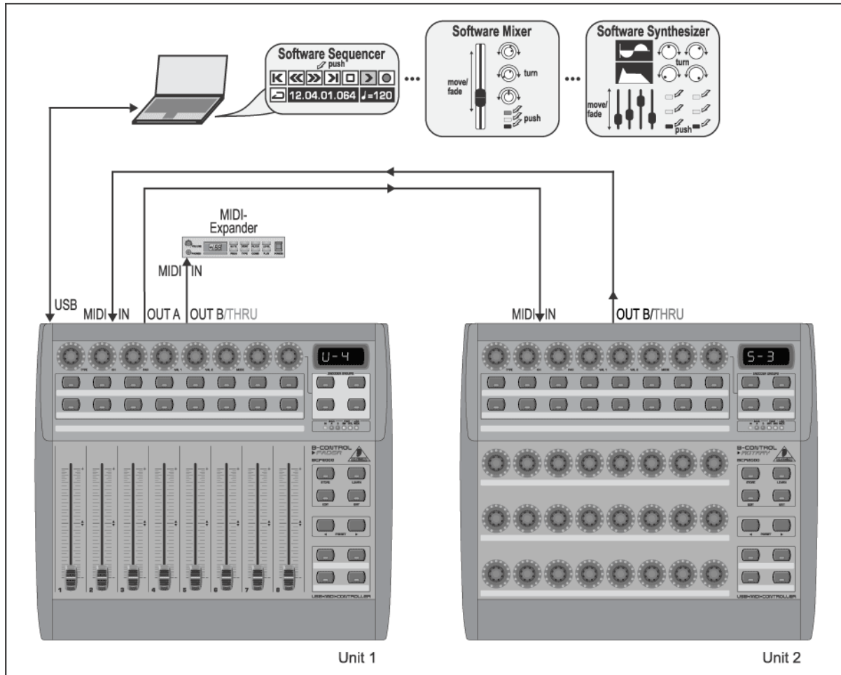
Fig. 4.4: Empleo en modo USB 4 (expandido)
