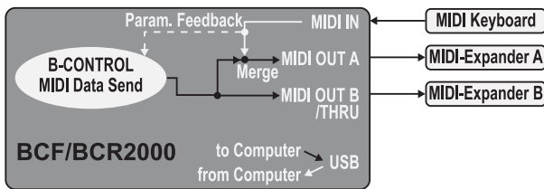
Fig. 4.8: Asignación y empleo en modo independiente 3
