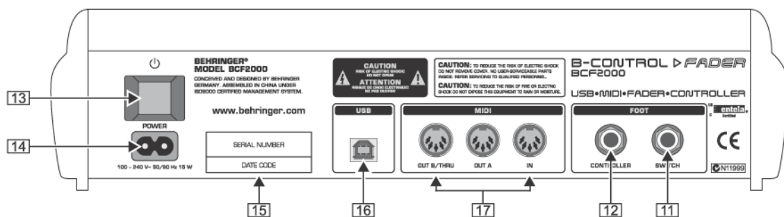
Fig. 3.2: La parte posterior del BCF2000 (los elementos de control 13 a 17 concuerdan con el BCF2000)
