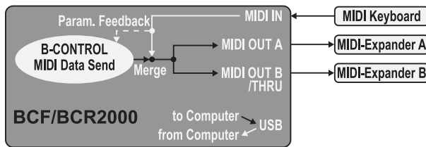
Fig. 4.6: Asignación y empleo en modo independiente 1
