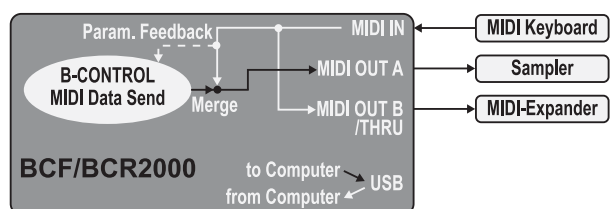
Fig. 4.7: Asignación y empleo en modo independiente 2
