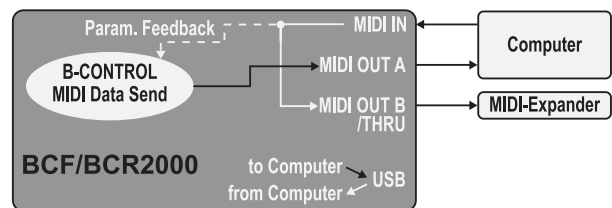
Fig. 4.9: Asignación y empleo en modo independiente 4
